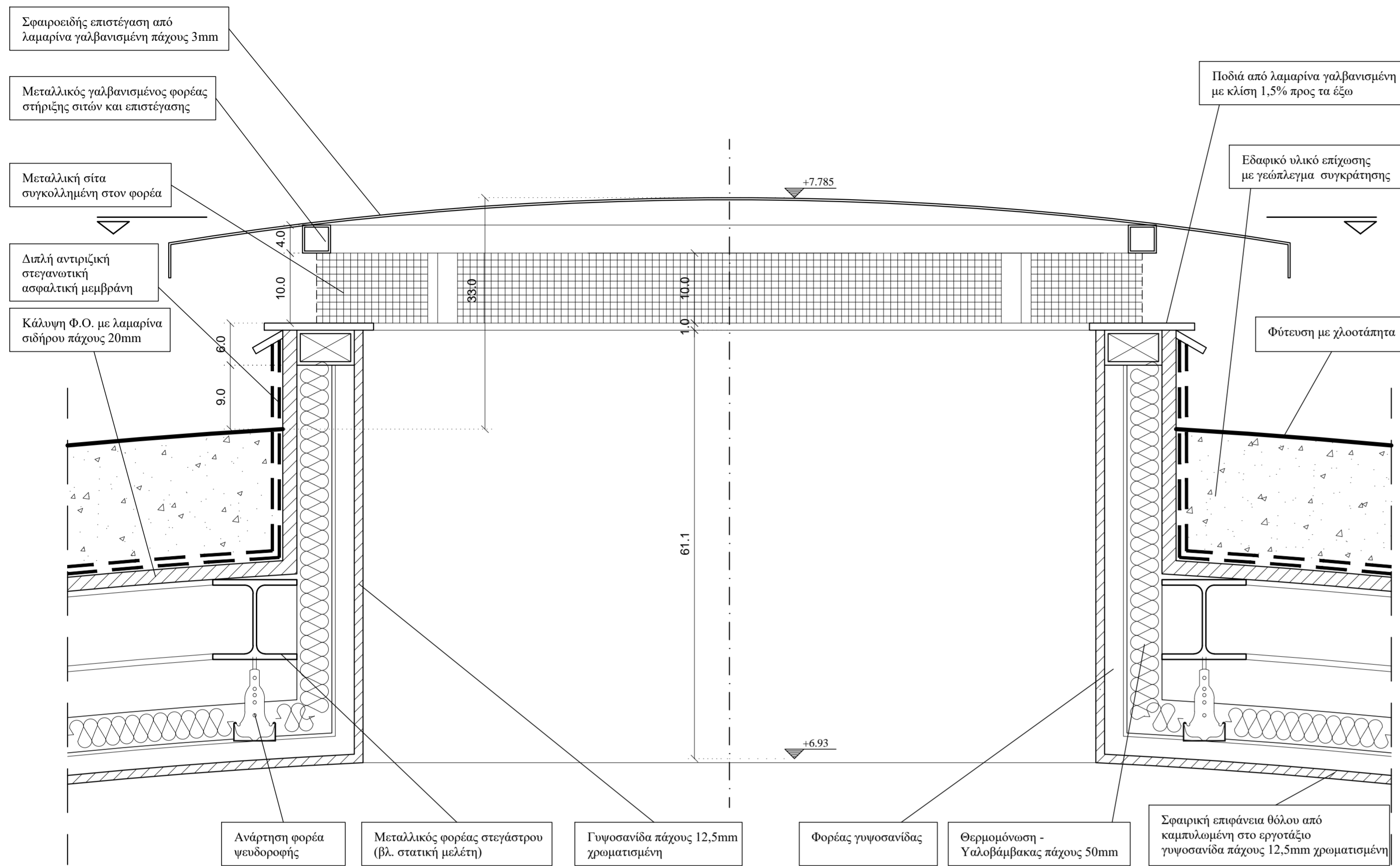
ΤΟΜΗ ΚΛΙΜΑΚΑ 1:5
