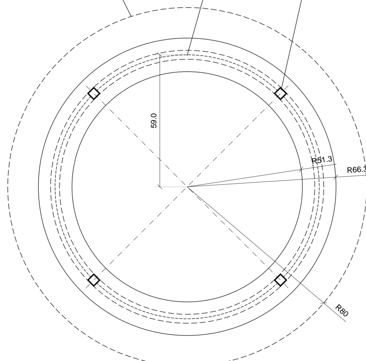
ΚΑΤΟΨΗ ΚΛΙΜΑΚΑ 1:10
